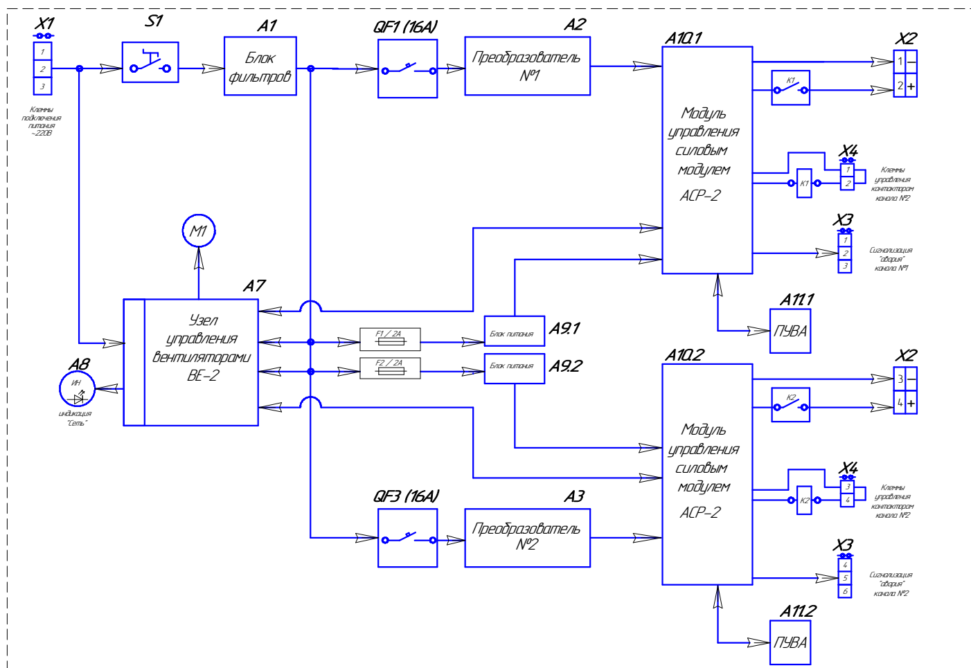
Схема структурная Агрегат BA2450/50
